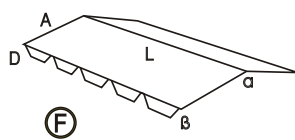
CUMEEIRA SHED LISA
