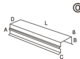
RUFO CHAPÉU LISO COM BITS
